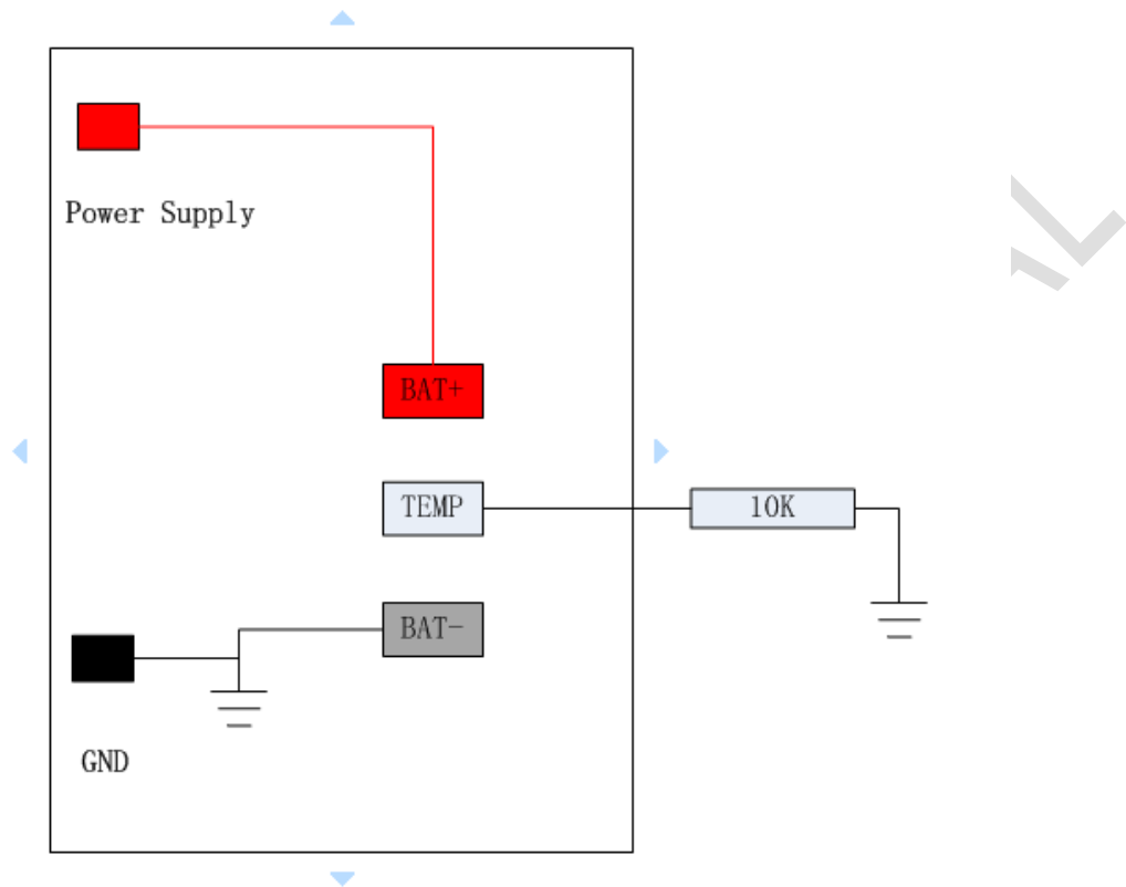
图 4.2 NTC 夹具接线方法
